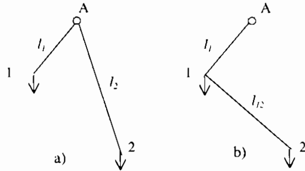
Hình 7.7. Sơ đồ hình tia(a) và sơ đồ liên thông (b).
