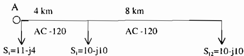
Hình 7.22. Sơ đồ xác định \Delta U_{\max} sự cố
