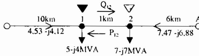
Hình 7.25. Sơ đồ cung cấp điện.
