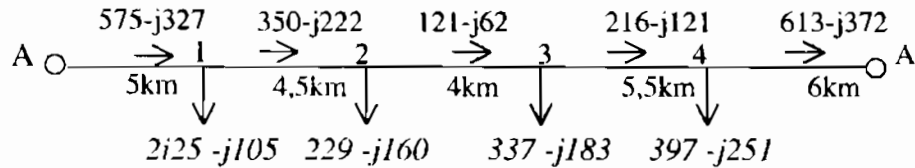
Hình 7.26. Sơ đồ mạng kín xác định phân bố công suất.
