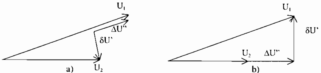
Hình 7.11. Các đồ thị vectơ của điện áp đầu và cuối đường dây.
