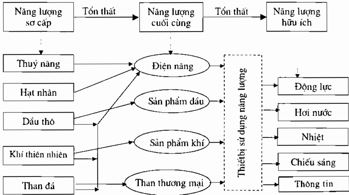
Hình 2.1. Hệ thống biến đổi và sử dụng năng lượng.
